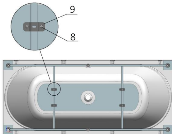
Рисунок 3а - Фиксация каркаса ванны
