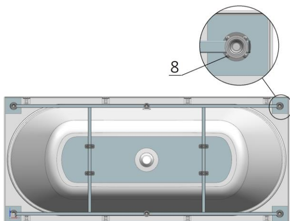
Рисунок 4а - Установка ножки
