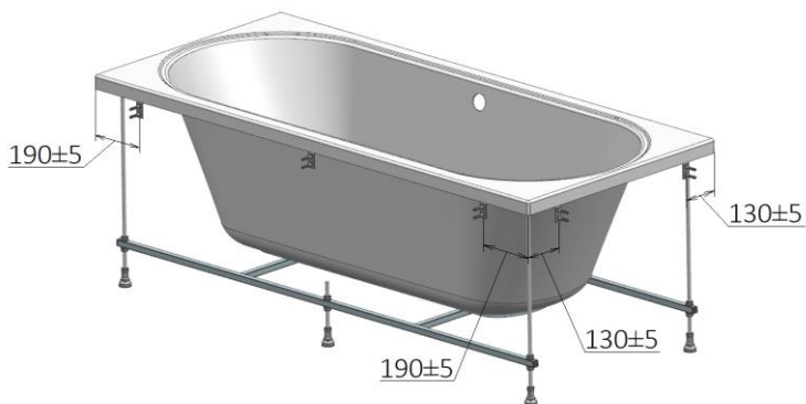
Рисунок 5а - Схема расположения креплений кронштейнов к стене
