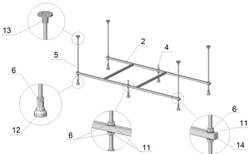
Рисунок 2а – Сборка каркаса ванны
