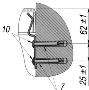
Рисунок 6а - Крепление ванны к стене
