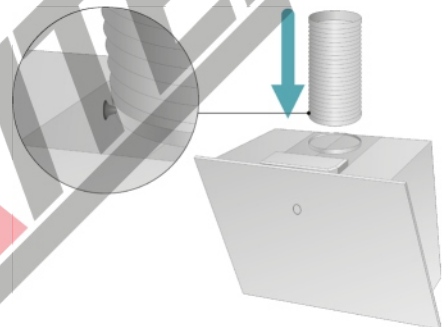
Рис.7 а. Подсоединения пластиковой гофры
