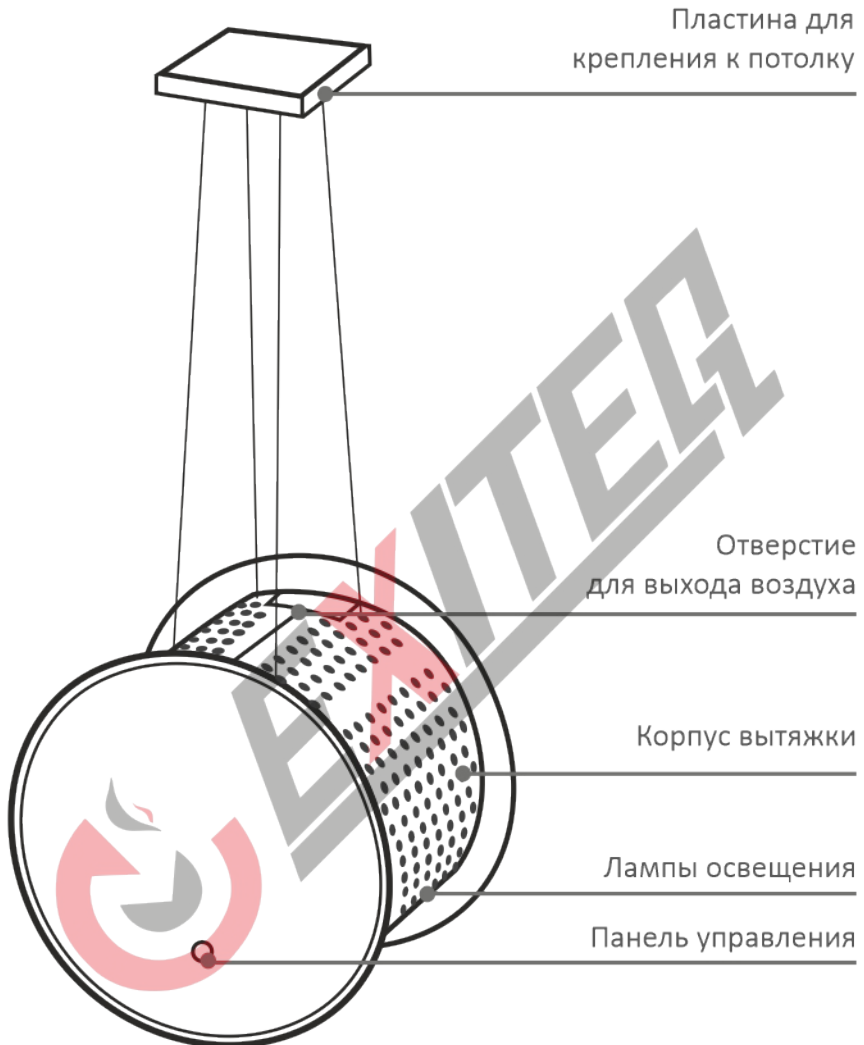
Рис.2 Наружная часть вытяжки состоит из следующих составных частей
